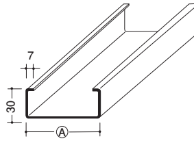
53-33 65補強材 A=65mm/高さ30mm/3m(在庫品)/t=1.2/1束50本入 取寄品 | A=40-45-50-75-90-100/高さ20mm
