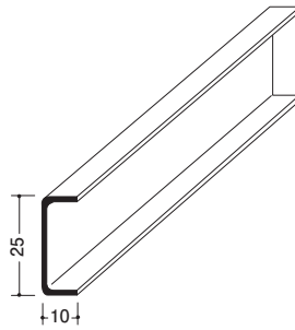
53-42 C25チャンネル(振れ止め用チャンネル) 3m(在庫品)/t=1.0/1束10本入 スタッド50-65-75-90-100mm用
