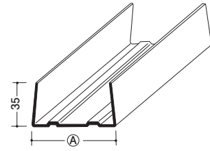
53-35 ランナー A=40mm/3m(在庫品)/t=0.6/1束4本入 A=45mm/3m(在庫品)/t=0.6/1束4本入 A=65mm/3m(在庫品)/t=0.6/1束4本入 取寄品 | A=50-75-90-100
