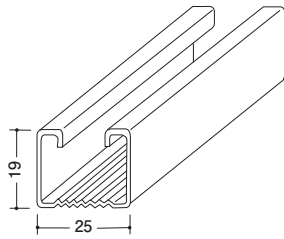
53-02 19Sバー 3m/t=0.35/1束20本入
