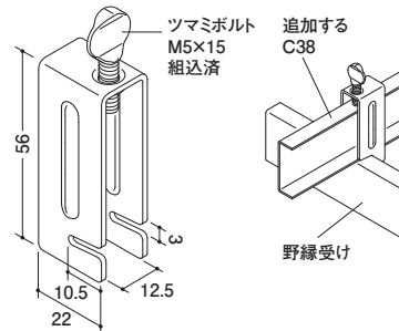
53-532 新クロス金具 500個入
