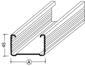
53-31 65スタッド A=65mm/3m(在庫品)/t=0.6/1束4本入 取寄品 | A=40-45-50-75-90-100
