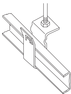
53-21 ミニハンガー C-19チャンネル用 H=33 C-25チャンネル用 H=37 C-38チャンネル用 H=50 天井裏が狭い場合 500入
