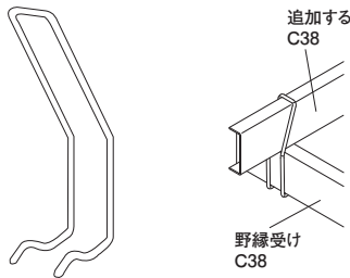
53-53 ワイヤークリップ(軽みぞ型取付金具) 100個入
