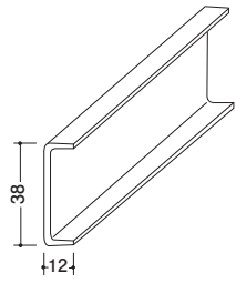
53-01 C38チャンネル 3m/t=1.0/1束10本入
