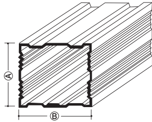
53-46 SQバー A×B=40×45/3m(在庫品)/t=0.45/1束5本入 A×B=45×65/3m(在庫品)/t=0.45/1束5本入 取寄品 | A×B=40×20-40×25 40×40-40×50
