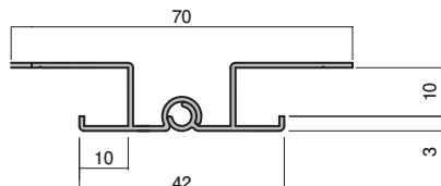
20-52 フリー入隅2型 3m / 10本入 角度自在の入隅(90°~180°)
