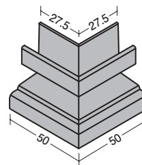
20-57 オールアルミ水切り出隅 5個入 水切りのコーナー部材
