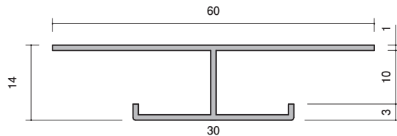
20-79 オールアルミジョイント 3m / 20本入 パネル同士のジョイント部材
