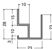
20-53 オールアルミ下がり壁露受け 3m / 10本入 下がり出隅の結露受け部材
