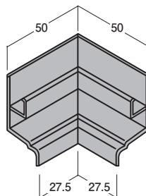
20-90 オールアルミ水切り入隅 5個入 水切りのコーナー部材
