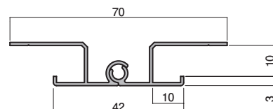
20-51 フリー出隅2型 3m / 10本入 角度自在の出隅(90°~180°)
