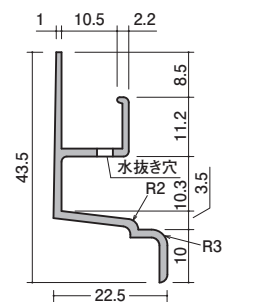
20-74 オールアルミ水切り 3m / 10本入 パネルと腰壁との縁切り部材
