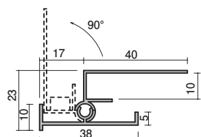
20-75 フリー廻り縁 3m / 10本入 角度自在の廻り縁(90°~180°) しかも結露も受ける部材
