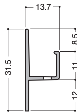
20-54 オールアルミカウンター見切 3m / 10本入 パネルとカウンターとの縁切り部材
