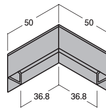
20-89 オールアルミカウンター見切入隅 5個入 カウンター見切のコーナー部材
