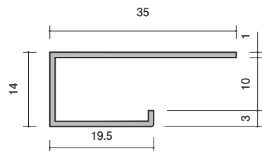
20-78 オールアルミ廻り縁 3m / 20本入 壁・天井の縁切り部材
