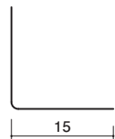
44-11 亜鉛アングル15 亜鉛メッキ鋼板/1820mm/t=0.27
