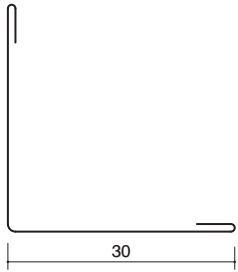
44-21 亜鉛アングル30内ハゼ付 亜鉛メッキ鋼板/1820mm/t=0.27
