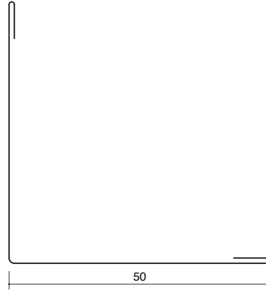
44-22 亜鉛アングル50内ハゼ付 亜鉛メッキ鋼板/1820mm/t=0.27
