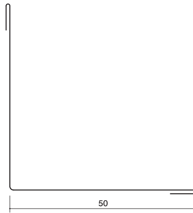
44-26 亜鉛アングル50外ハゼ付 亜鉛メッキ鋼板/1820mm/t=0.27
