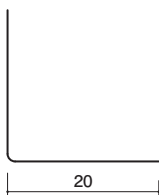
44-12 亜鉛アングル20 亜鉛メッキ鋼板/1820mm/t=0.27
