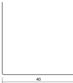
44-14 亜鉛アングル40 亜鉛メッキ鋼板/1820mm/t=0.27
