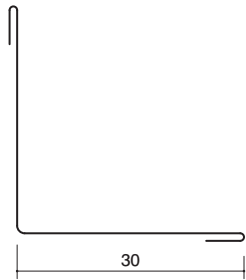
44-25 亜鉛アングル30外ハゼ付 亜鉛メッキ鋼板/1820mm/t=0.27
