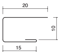
42-05 コ型ハゼ付9 亜鉛メッキ鋼板/1820mm/t=0.27
