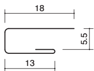
42-02 コ型ハゼ付5 亜鉛メッキ鋼板/1820mm/t=0.27
