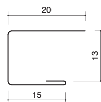
42-06 コ型ハゼ付12 亜鉛メッキ鋼板/1820mm/t=0.27
