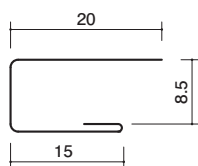
42-04 コ型ハゼ付8 亜鉛メッキ鋼板/1820mm/t=0.27
