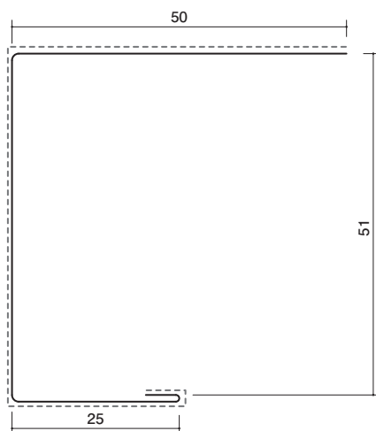
44-86 カラー鉄板コ型50 1820mm/クリアム/t=0.27
