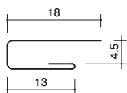
42-01 コ型ハゼ付4 亜鉛メッキ鋼板/1820mm/t=0.27
