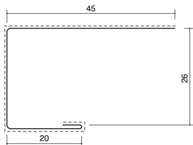
44-85 カラー鉄板コ型25 1820mm/クリアム/t=0.27
