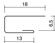
42-03 コ型ハゼ付6 亜鉛メッキ鋼板/1820mm/t=0.27
