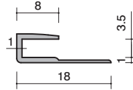
37-01 アルミ 3.5コS 1820mm-2420mm-2730mm アルマイトシルバー
