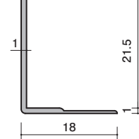
39-21 アルミ 21.5コS 2730mm アルマイトシルバー
