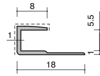
37-03W アルミ 5.5コS ホワイト 2730mm/ホワイト(焼付塗装)
