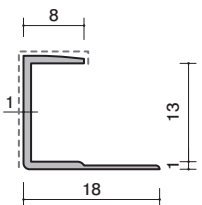
37-08W アルミ 12.5コS ホワイト 2730mm/ホワイト(焼付塗装)
