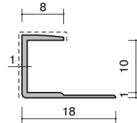
37-06W アルミ 9.5コS ホワイト 2730mm/ホワイト(焼付塗装)
