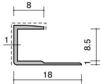
37-05W アルミ 8.5コS ホワイト 2730mm/ホワイト(焼付塗装)
