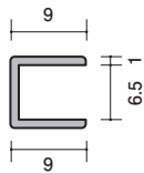
39-00 アルミ CCAL-6.5 3000mm/アルマイトシルバー
