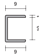
39-01 アルミ CCAL-9.5 3000mm/アルマイトシルバー
