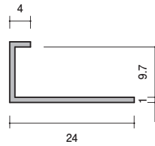
31-09 アルミ C-497 3000mm/アルマイトシルバー
