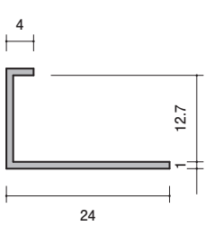
31-10 アルミ C-4127 3000mm/アルマイトシルバー
