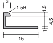
39-42 アルミ CAG-4.5 2730mm/アルマイトシルバー
