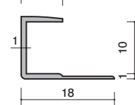
37-06 アルミ 9.5コS 1820mm-2730mm アルマイトシルバー
