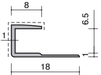
37-04W アルミ 6.5コS ホワイト 2730mm/ホワイト(焼付塗装)
