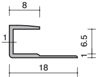
37-04 アルミ 6.5コS 1820mm-2420mm-2730mm アルマイトシルバー
