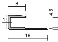
37-02W アルミ 4.5コS ホワイト 2730mm/ホワイト(焼付塗装)
