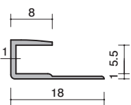
37-03 アルミ 5.5コS 1820mm-2730mm アルマイトシルバー
