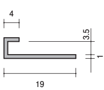
34-19 アルミ C-435 3000mm/アルマイトシルバー
