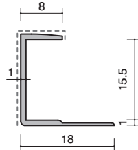
37-99W アルミ 15.5コS ホワイト 2730mm/ホワイト(焼付塗装)
