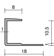
37-07 アルミ 10.5コS 1820mm-2730mm アルマイトシルバー
