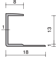
37-08 アルミ 12.5コS 1820mm-2730mm アルマイトシルバー
