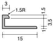
39-41 アルミ CAG-3.5 2730mm/アルマイトシルバー
