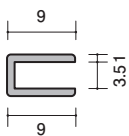
39-19 アルミ CCAL-3.5 3000mm/アルマイトシルバー
