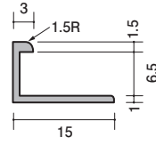
39-43 アルミ CAG-6.5 2730mm/アルマイトシルバー
