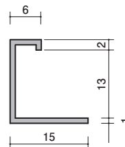
33-88 アルミ AEC-613 3000mm/アルマイトシルバー
