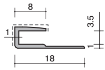
37-01W アルミ 3.5コS ホワイト 2730mm/ホワイト(焼付塗装)
