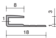
39-20 アルミ 3.0コS 2730mm アルマイトシルバー
