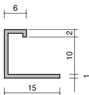
33-87 アルミ AEC-610 3000mm/アルマイトシルバー
