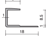
37-05 アルミ 8.5コS 1820mm-2730mm アルマイトシルバー
