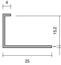
31-29 アルミ C-4152 3000mm/アルマイトシルバー
