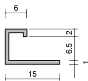
33-86 アルミ AEC-606 3000mm/アルマイトシルバー
